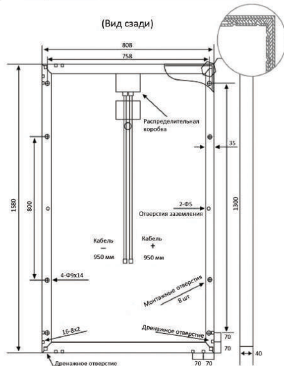
Солнечный модуль Sunspare TDM200-A-72
