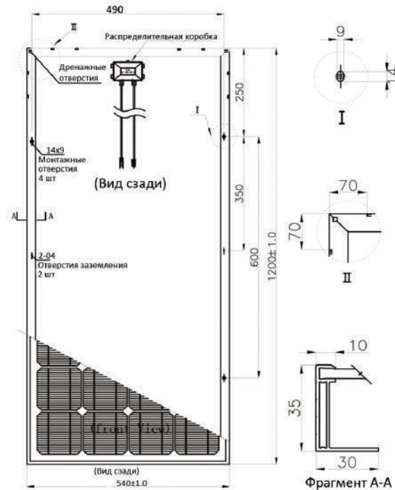
Солнечный модуль Sunspare GPM100W36
