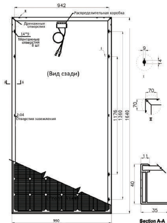
Солнечный модуль Sunspare TDM250-B-60
